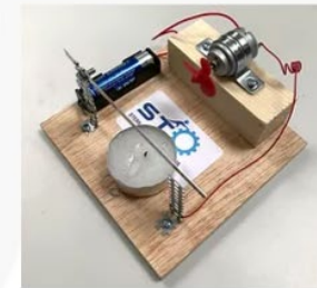
Ventilator met bimetaal
